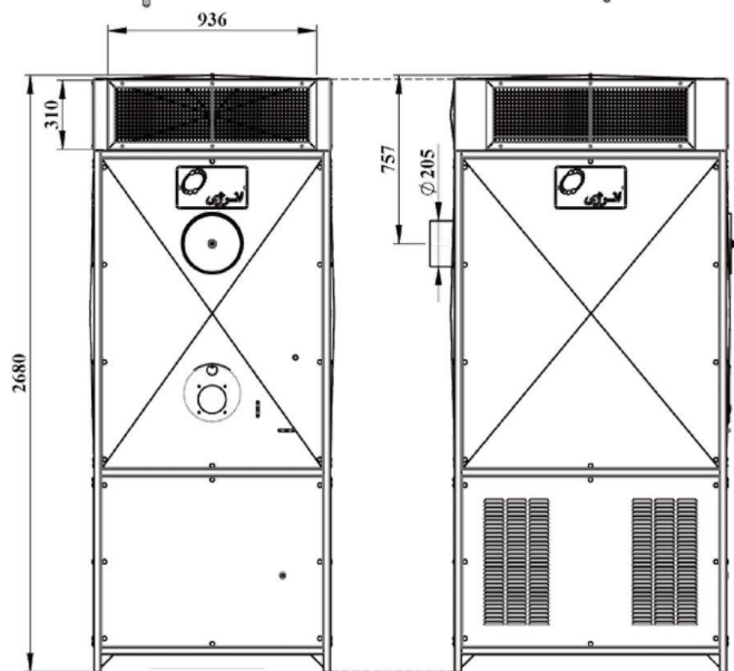
نمای روبرو
