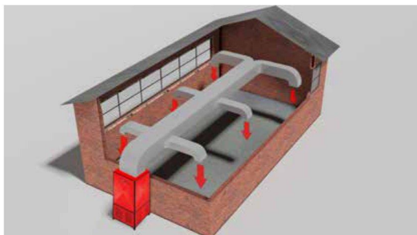
شکل (۸) نصب کوره در خارج از سالن
