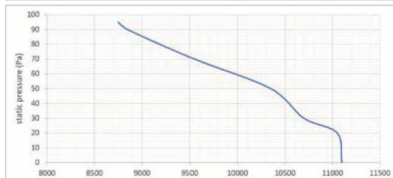
نمودار ۱ - نمودار هواهی- افت فشار
