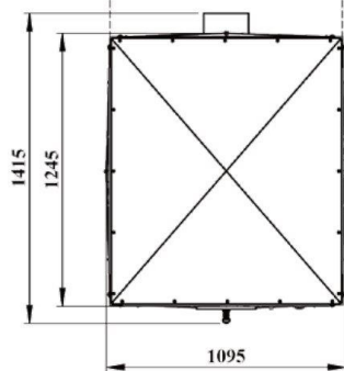
نمای بالا
